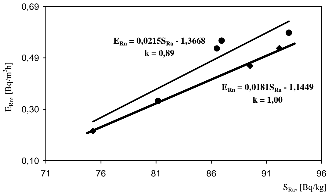
Rys.3. Zależność efektywności ekshalacji radonu E_{Rn} od stężenia radu S_{Ra} .
